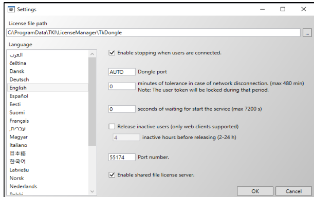
图 6: 设置对话框
