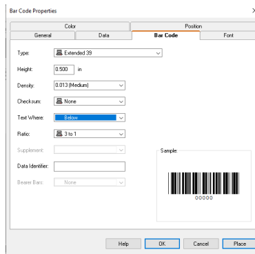
图15 条形码页
