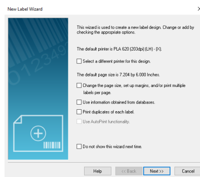
图2 新标签向导
