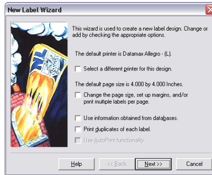
图 2 新标签向导
