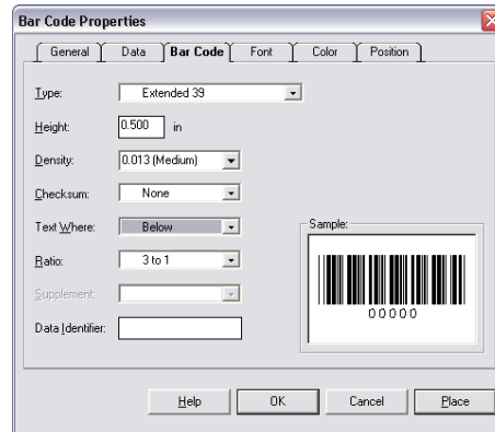
图 15 条形码页
