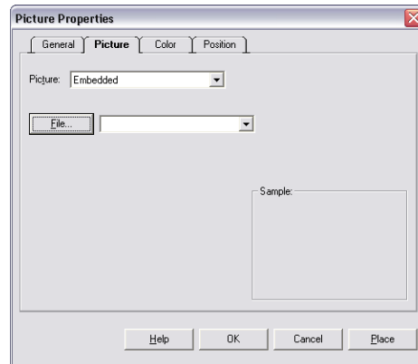
图 5 图片页
