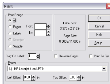
图 19 打印属性
