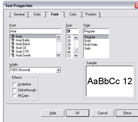
图 7 字体页
