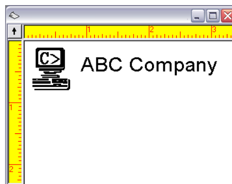
图 8 添加文本
